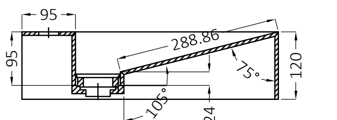
SECCIÓN A-A'
