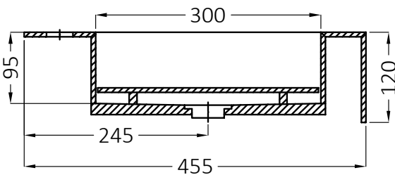
SECCIÓN A-A'
