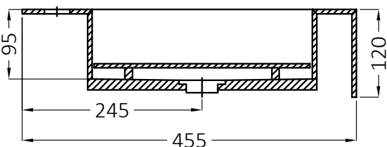
SECCIÓN A-A'
