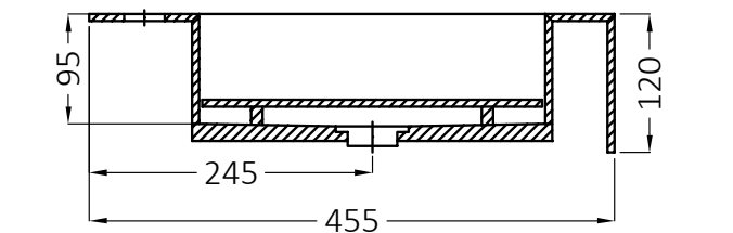
SECCIÓN A-A'
